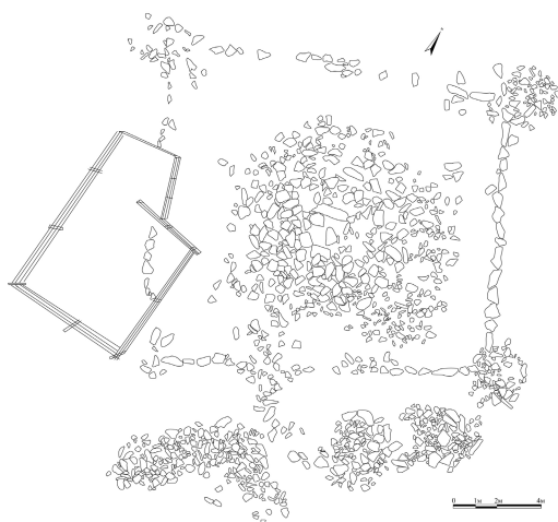
Зураг 16. Дурсгал-14. Хиргисүүрийн дэвсгэр зураг
