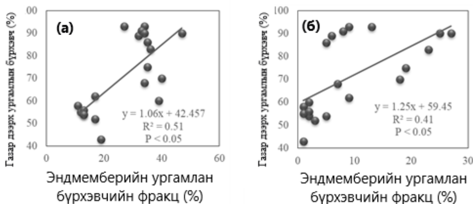
Зураг 4. (a) Ландсат 8 болон (b) Сентинел 2 хиймэл дагуулаас авсан зураг дахь пикселүүдийг үл холих аргаар тооцсон эндмемберийн ургамлан бүрхэвчийн фракц (VGT)-тай Харденберг нар (2001)-ын аргачлалын дагуу (томьёо 1, 2) хээрийн хэмжилтээр тооцсон ургамлан бүрхэвчийг харьцуулсан үр дүн.
