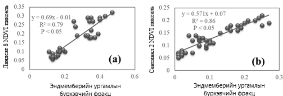
Зураг 3. (a) Ландсат 8 болон (b) Сентинел 2 хиймэл дагуулаас авсан зураг дахь пикселийн ургамлын өөрчлөлтийн нормчилсон индекс (NDVI) ба мөн энэ пикселүүдийг үл холих аргаар тооцсон эндмемберийн ургамлын бүрхэвчийн фракц (VGT)-ийг харьцуулсан үр дүн.
