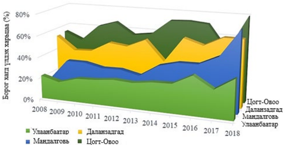
Зураг 2. Ургамлын борог хагд үлдэгдлийн түвшин (3-р тэгшитгэлээс тооцоолсон) (зураг дээр үсгээр хийсэн тэмдэглэгээний тайлбарыг дараах байдлаар ашиглана уу: Улаанбаатар-UB; Мандалговь-MG; Даланзадгал-DZ; Цогт-Овоо-TO; Ratio (%)- Борог хагдны хувь).
