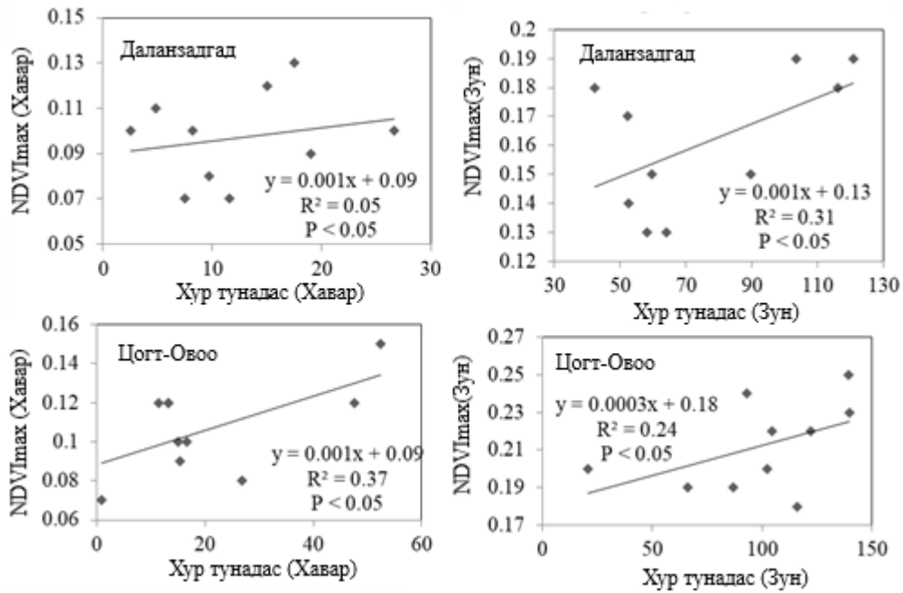
Зураг 1. 2007-2016 оны хоорондох хамгийн их ургамлын өөрчлөлтийн нормчилсон индекс (NDVI) ба хур тунадасны хоорондох хамаарал NDVI max - хамгийн их ургамлын өөрчлөлтийн нормчилсон индекс, \Sigma Precipitation- Нийлбэр хур тунадас)
